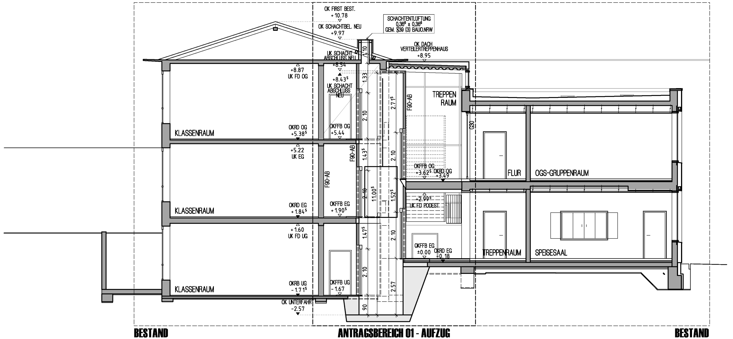
SCHNITT A-A
