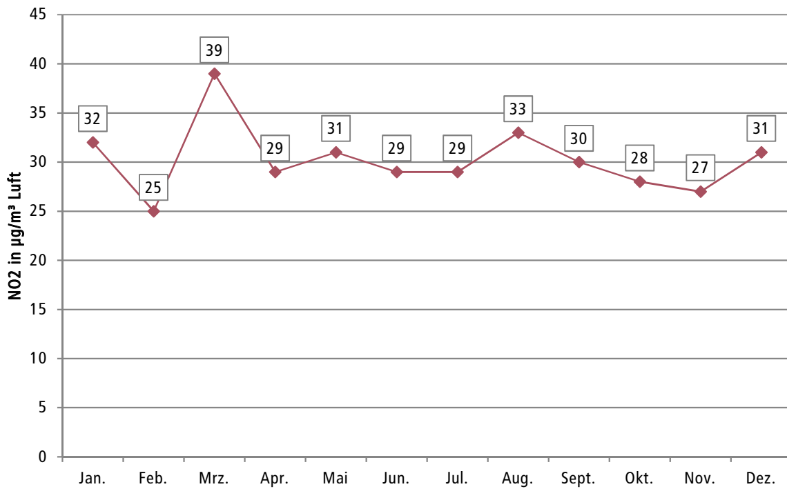
Abbildung 20: Stickstoffdioxid (NO 2 ) Aachen (in µg/m 3 Luft) im Jahr 2022; Messstation am Verkehrsknotenpunkt Wilhelmstraße. © Stadt Aachen FB02/200
