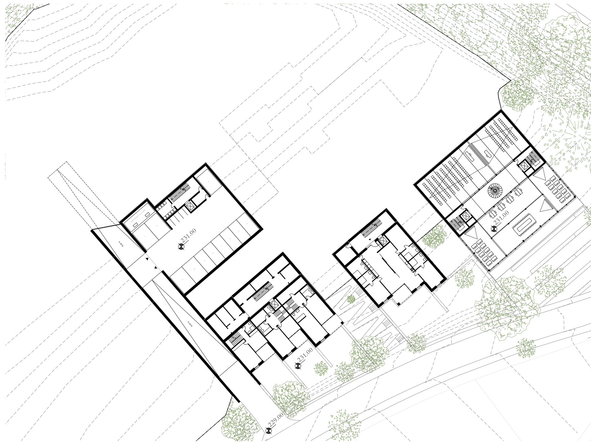
Grundriss Ebene 02, EG M 1/500
