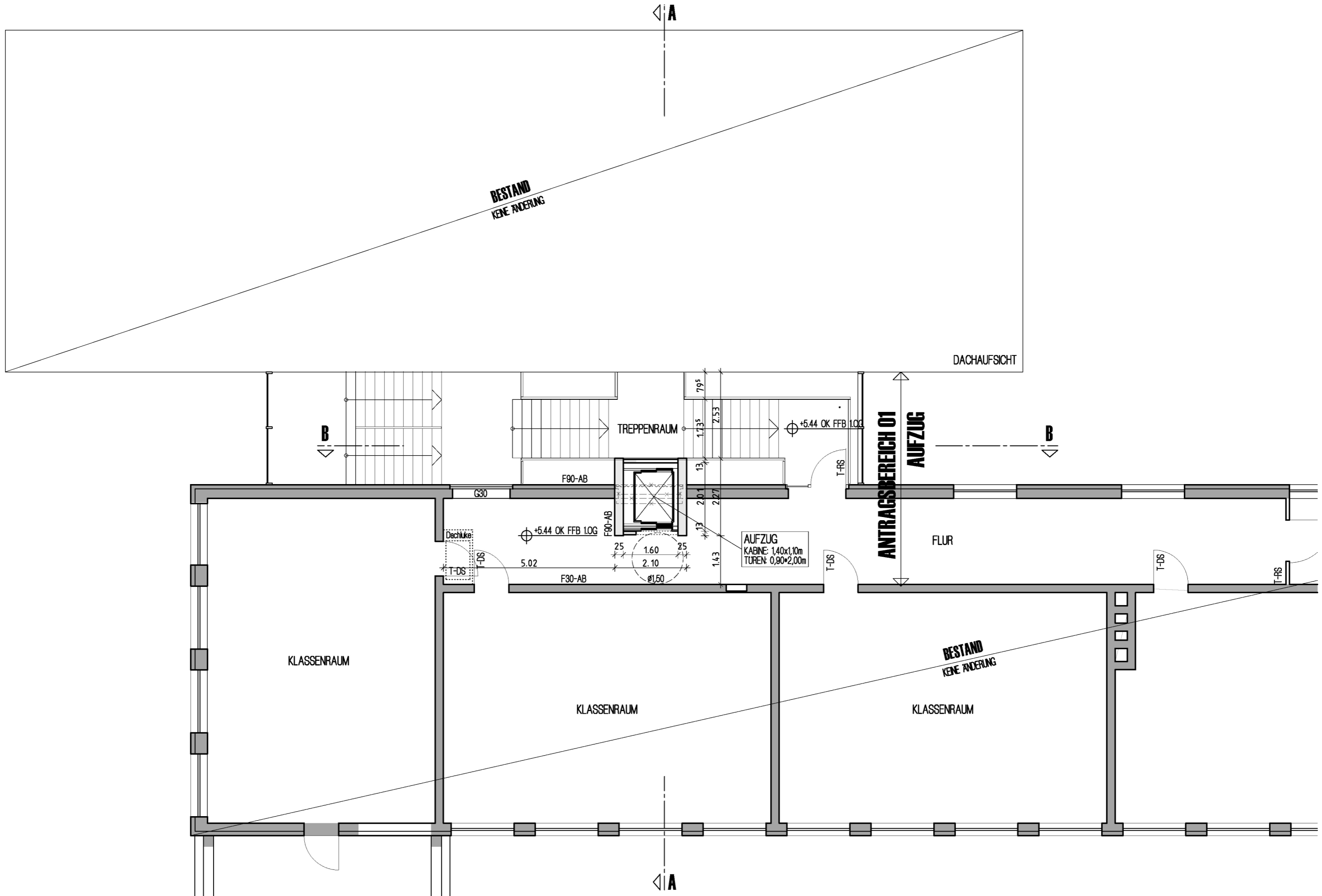
GRUNDRISS OBERGESCHOSS
