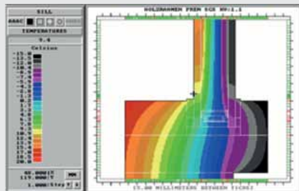
Abstandhalter als warme Kante (Kunststoff od. V2A)
