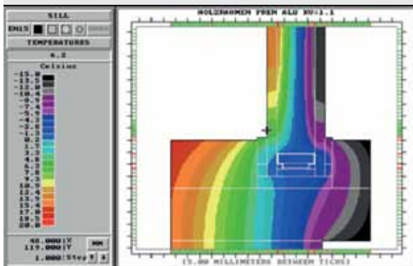
Abstandhalter aus Aluminium
