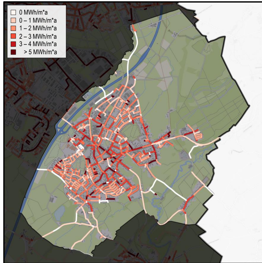
Wärmeliniendichte
