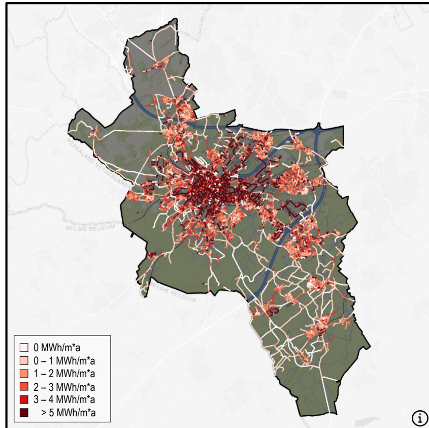
Wärmeliniendichte
