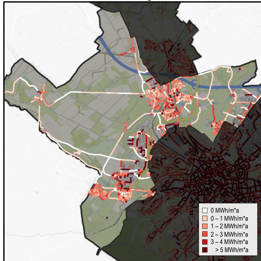
Wärmelinienichte Ausschnitt Laurensberg
